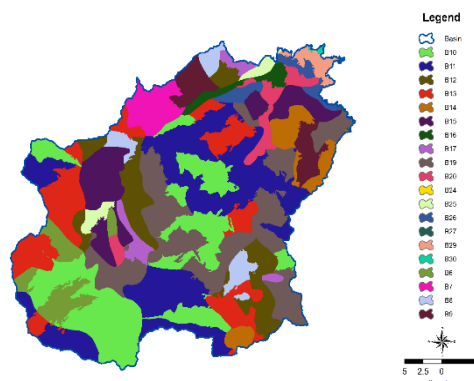
شکل ۵- نقشه خاک حوزه باراندوزچای Figure 5. Soil map of the Barandouz Chay basin
