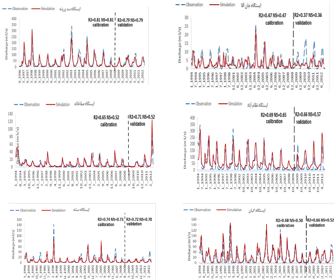
شکل ۲- نتایج واسنجی و صحت‌سنجی دبی ایستگاه‌های مختلف و نیترات کل حوزه زرنه‌رود در ماه‌های مختلف سال Figure 2. Calibration and Validation Results of Different Stations and Total Nitrate of Zarinerood Basin
