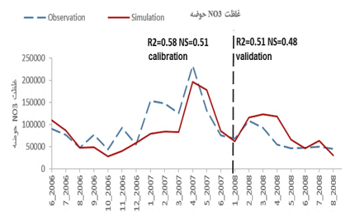
شکل ۲- نتایج واسنجی و صحت‌سنجی دبی ایستگاه‌های مختلف و نیترات کل حوزه زرينه‌رود در ماه‌های مختلف سال Figure 2. Calibration and Validation Results of Different Stations and Total Nitrate of Zarinerood Basin
