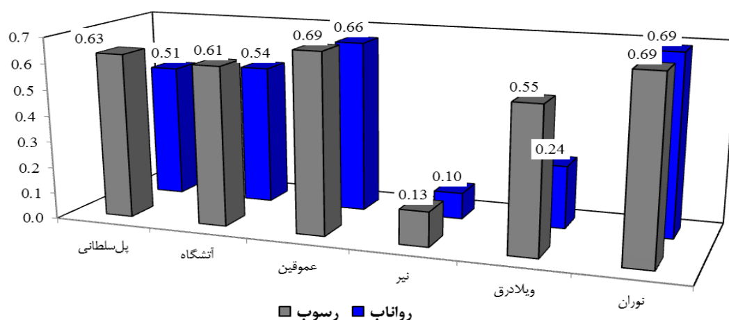
شکل ۴- ضریب تغییرات مقادیر رواناب و رسوب در ایستگاه‌های آبخیز مورد مطالعه
