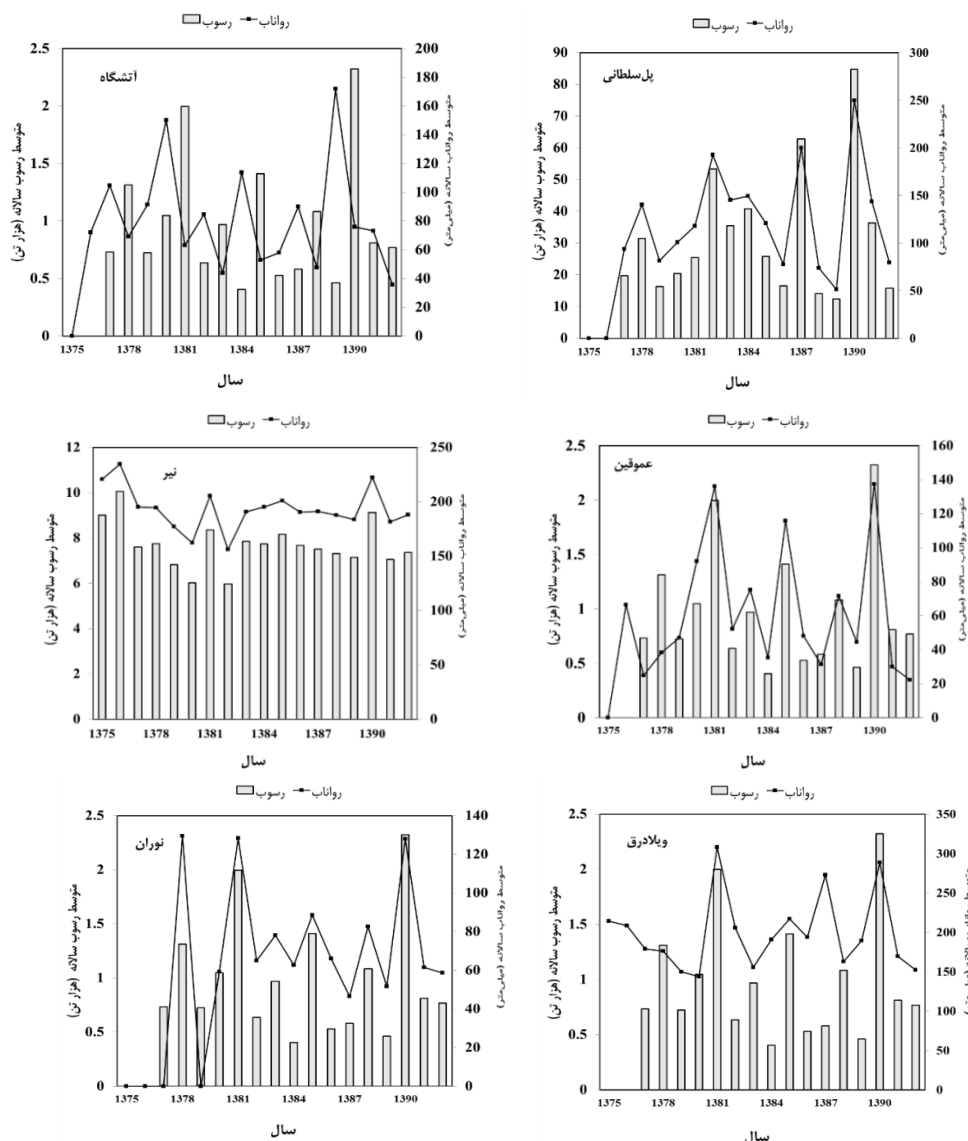
شکل ۵- تغییرات مقادیر رواناب و رسوب در طول دوره آماری موجود در ایستگاه‌های هیدرومتری مورد مطالعه استان اردبیل
