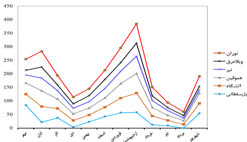
شکل ۲- توزیع بارش‌های ماهانه در ایستگاه‌های مورد مطالعه (۱۳۷۵-۹۲) Figure 2. Distribution of monthly precipitation in the studied stations (1996-2013)
