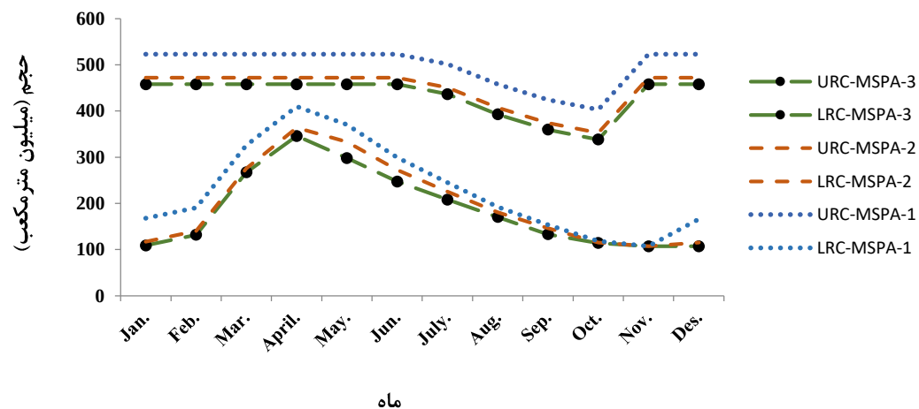
شکل ۴- منحنی فرمان سد زرینه‌رود بر اساس MSPA با داده‌های تاریخی (۱۳۸۷-۲۰۱۸) Figure 4. Zarrinehroud Dam rule curve based MSPA with historical data (1987-2018)
