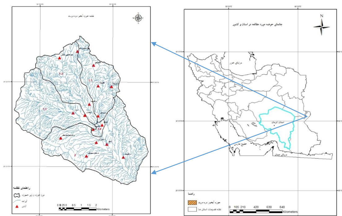
شکل ۱- موقعیت آبخیز دره مرید (محل مطالعه) در استان کرمان Figure1. The Location of Darreh Morid Watershed (the study area) in Kerman Province
