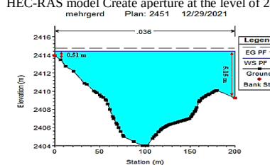
شکل ۱۵- فاصله ۲۲۰۰ متری از مقطع سد در مدل HEC-RAS ایجاد روزنه در تراز ۲۴۵۱
