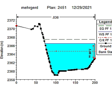
شکل ۱۹- فاصله ۴۷۰۰ متری از مقطع سد در مدل HEC-RAS ایجاد روزنه در تراز ۲۴۵۱
