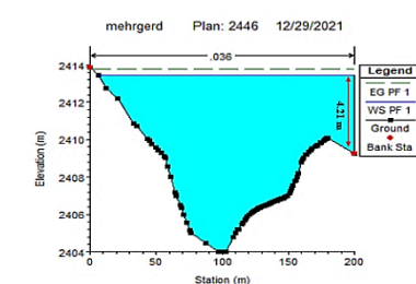
شکل ۹- فاصله ۲۲۰۰ متری مقطع سد در مدل HEC-RAS ایجاد روزنه در تراز ۲۴۴۶
