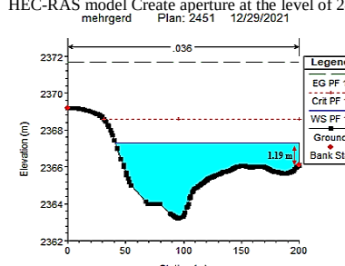
شکل ۱۸- فاصله ۴۴۰۰ متری از مقطع سد در مدل HEC-RAS ایجاد روزنه در تراز ۲۴۵۱
