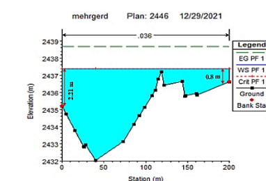
شکل ۸- فاصله ۳۰۰ متری مقطع سد در مدل HEC-RAS ایجاد روزنه در تراز ۲۴۴۶
