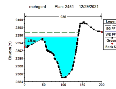
شکل ۱۷- فاصله ۳۱۰۰ متری از مقطع سد در مدل HEC-RAS ایجاد روزنه در تراز ۲۴۵۱
