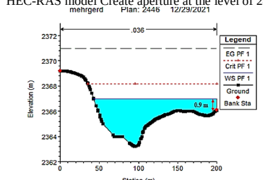
شکل ۱۲- فاصله ۴۴۰۰ متری از مقطع سد در مدل HEC-RAS ایجاد روزنه در تراز ۲۴۴۶
