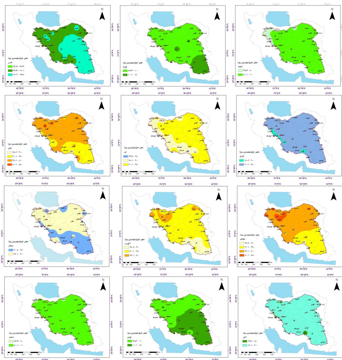
شکل ۳- برآورد مقادیر تبخیر و تعرق پتانسیل در آبخیز مرکزی در افق آینده میانی (۲۰۴۱-۲۰۶۰) Figure 3. Estimation of potential evapotranspiration values in the central Iran watershed in the middle future horizon (2041-2060)
