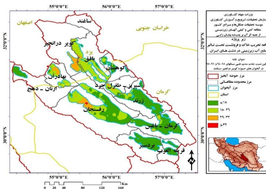
شکل ۴- نقشه پهنه‌بندی مقادیر میانگین پارامتر نسبت جذب سدیم منابع آب زیرزمینی حوزه آبریز درانجیر Figure 4. The zoning map of the mean values of the sodium absorption ratio parameter of groundwater resources in the Daranjir watershed
