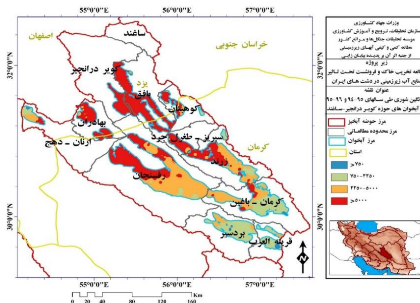
شکل ۳- نقشه پهنه‌بندی مقادیر میانگین پارامتر هدایت الکتریکی منابع آب زیرزمینی حوزه آبریز درانجیر Figure 3. The zoning map of the mean values of electrical conductivity parameter of groundwater resources in the Daranjir watershed
