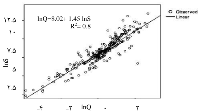
شکل ۸- رابطه خطی بر اساس لگاریتم دبی جریان و رسوب معلق در ایستگاه حاجی قوشان
