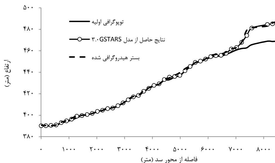
شکل ۸- پروفیل طولی رسوبگذاری مخزن شهید رجایی بعد از گذشت ده سال از زمان بهره برداری
