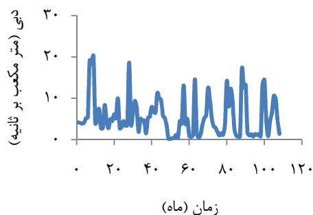
شکل ۷- تغییرات دبی جریان در شاخه شیرین رود
