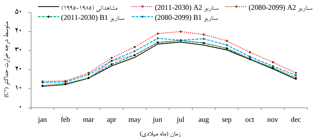
شکل ۳- الگوی تغییرات میانگین حداکثر درجه حرارت ماهانه حوزه آبخیز قزاقلی برای دوره آتی و دوره مشاهداتی تحت دو سناریو A2 و B1
