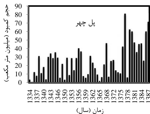
شکل ۲- حجم کمبود برای کل ایستگاه‌ها در حد آستانه Q_7 .
