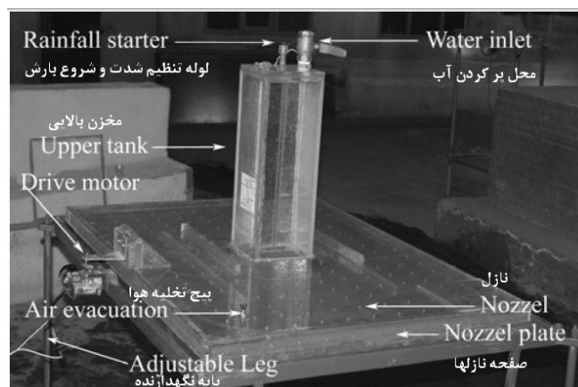
شکل ۵- بخش‌های تشکیل دهنده دستگاه شبیه ساز باران (وهاپی و نیک کامی، ۱۳۸۷)
