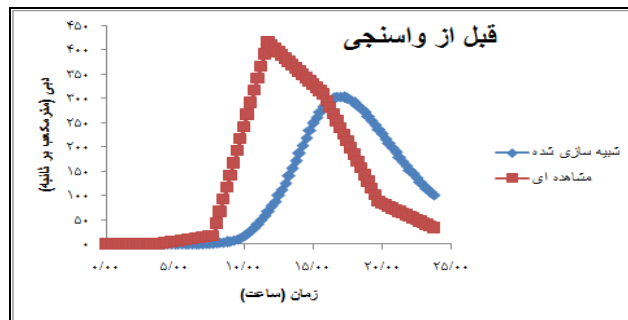
شکل (۴-۱۹) سیلاب مورخ ۱۳۷۶/۰۹/۲۳ قبل از واسنجی.
