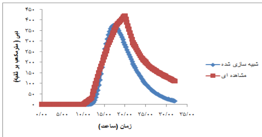
شکل ۵- آبنمود مشاهده‌ای و شبیه‌سازی شده برای اعتبارسنجی مدل در تاریخ 1378/11/25 .
