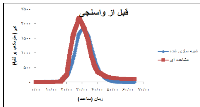
شکل (۴-۲۱) سیلاب مورخ ۱۳۷۳/۰۸/۲۵ قبل از واسنجی.
