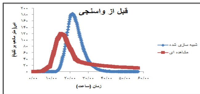
شکل (۴-۱۷) سیلاب مورخ ۱۳۶۹/۱۰/۱۲ قبل از واسنجی.
