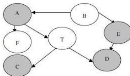
شکل ۲- نمایش گراف مستقیم و چرخه‌ای شبکه بیزین Figure2. The view of direct and cyclic Bayesian network
