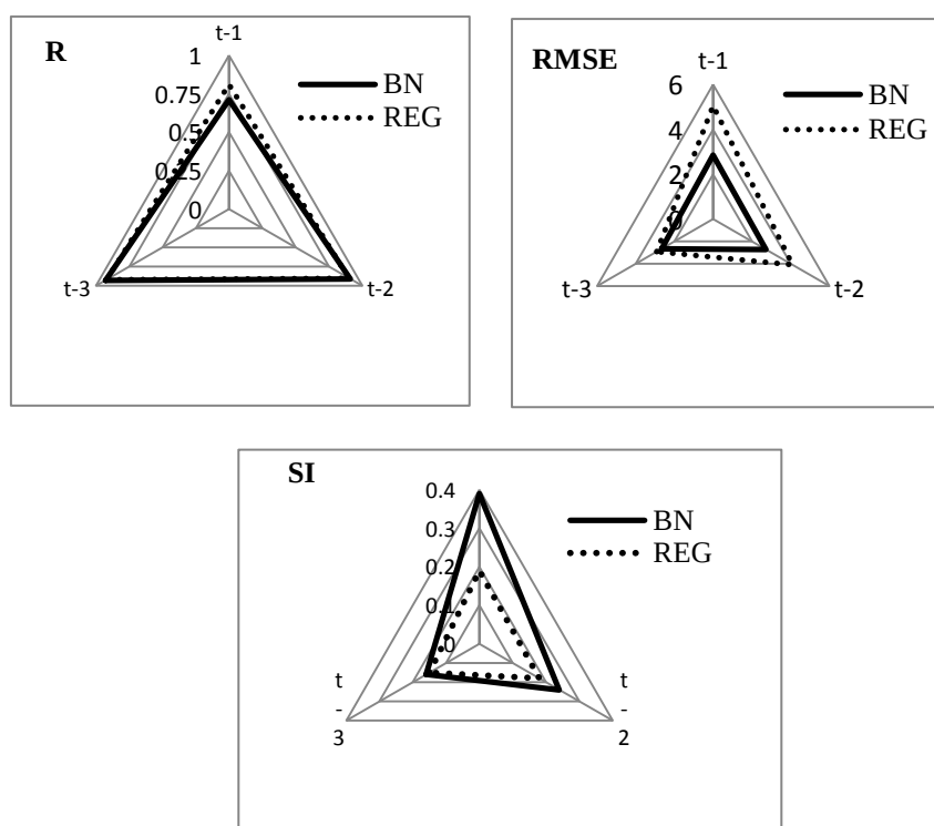
شکل ۵- عملکرد مدل شبکه بیزین و رگرسیون چند متغیره در مرحله تست برای پیش‌بینی دما ایستگاه سینوپتیک تبریز Figure 5. The performance of Bayesian network and multivariate linear regression in the testing for predicted temperature in Tabriz synoptic station
