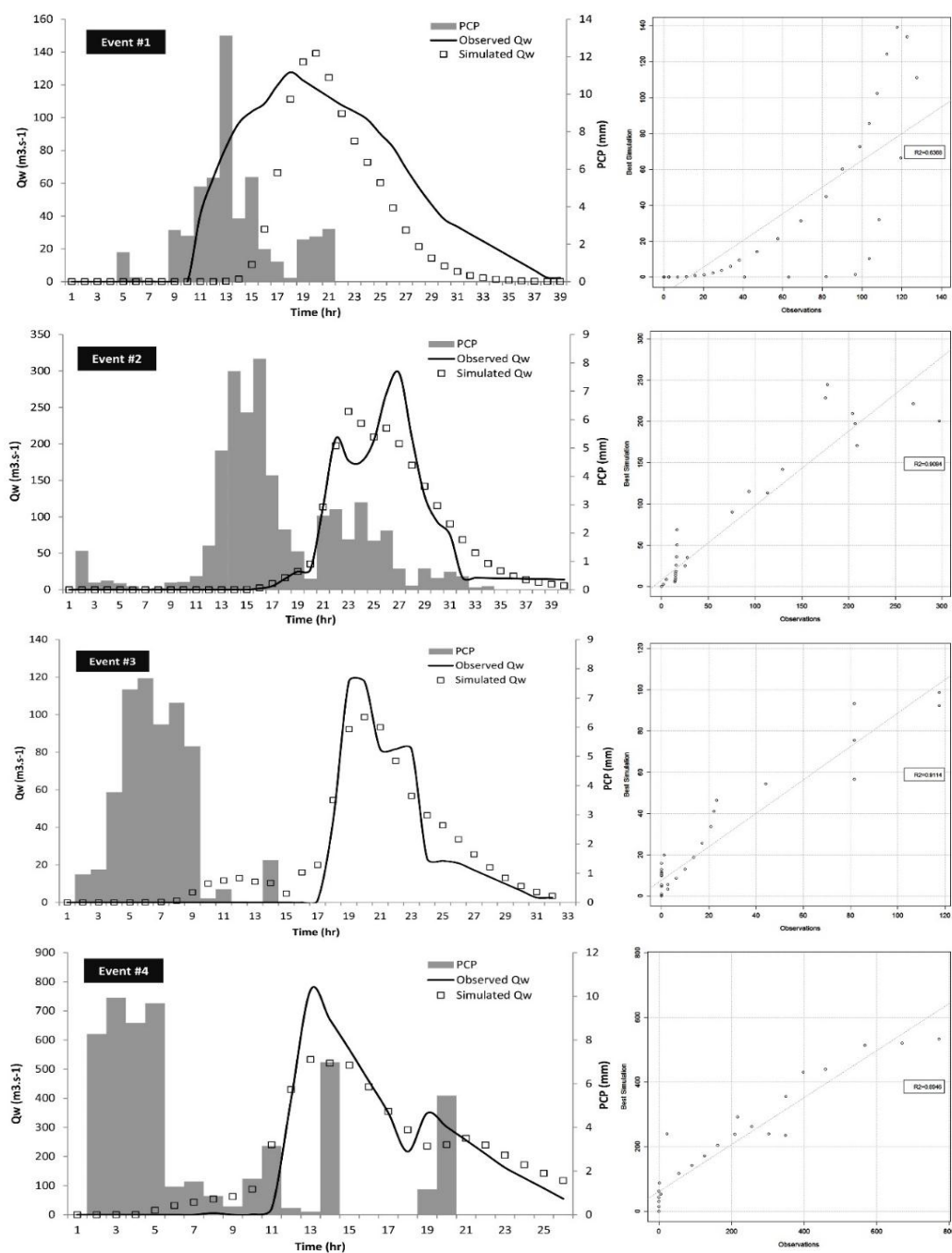
شکل ۳- دبی شبیه‌سازی شده ( Q_w Simulated) در برابر دبی مشاهده‌ای ( Q_w Observed) همراه با هیئوگراف بارش (PCP) بر اساس وقایع مختلف رگباری
