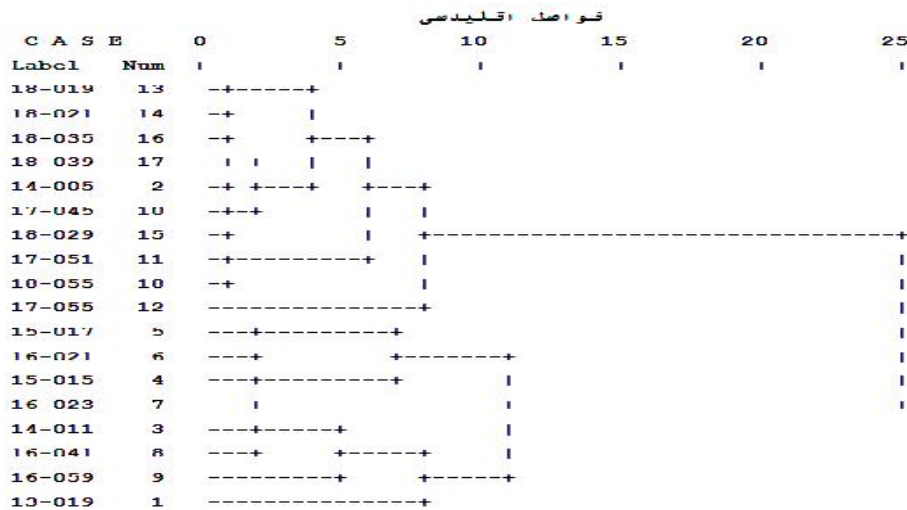
شکل ۳- نمودار خوشه‌ای زیرحوزه‌های همگن بر اساس عوامل مستقل Figure 3. Dendrogram of homogeneity catchments based of independent factors
