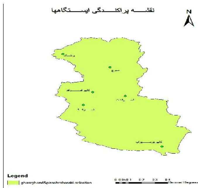
شکل ۲- نقشه پراکندگی ایستگاه‌های حوزه آبخیز رودخانه کاجو در استان سیستان و بلوچستان Figure 2. Distribution map of stations of watershed of river of Kajou in province of sistān & balouchestan
