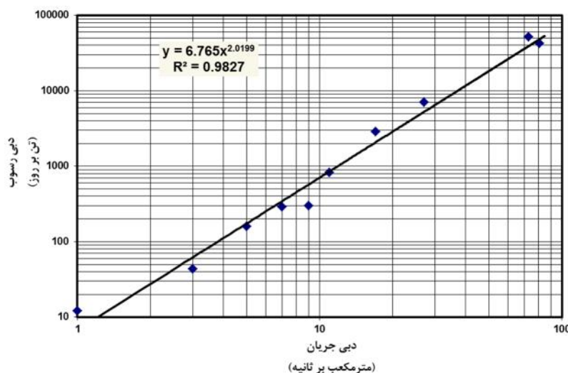
شکل ۴- منحنی سنجه حدوسط دسته‌ها مربوط به ایستگاه شیرگاه Figure 4. Logged mean loads sediment rating curve at Shirgah station
