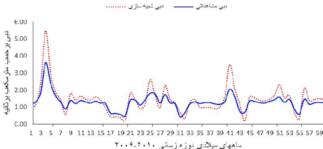
شکل ۴- مقایسه هیدروگراف‌های شبیه‌سازی شده و مشاهداتی در دوره اعتبارسنجی با پایه زمانی ماهانه
