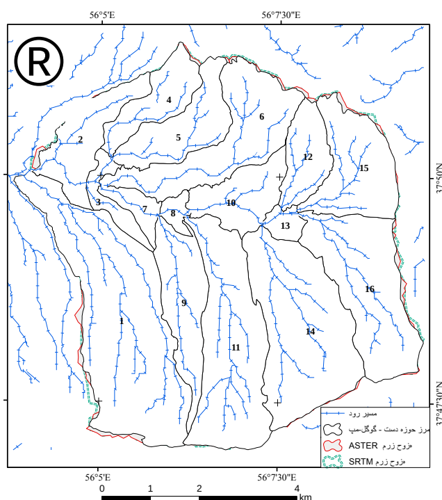
شکل ۴- مرز حوزه آبخیز یک‌چنار-اترک در محیط نرم‌افزار به‌صورت روش دستی (گوگل-ارث) و مدل خودکار Figure 4. The boundary of Yekechenar Watershed by manual method (based on Google Earth) and automated modeling
