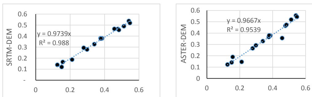
شکل ۵- انطباق میزان نسبت تحویل رسوب مدل خودکار (محور عمودی) با نسبت تحویل رسوب مدل دستی با استفاده از گوگل ارث (محور افقی): خط نقطه‌چین، خط رگرسیون بین آن‌ها را نشان می‌دهد.
