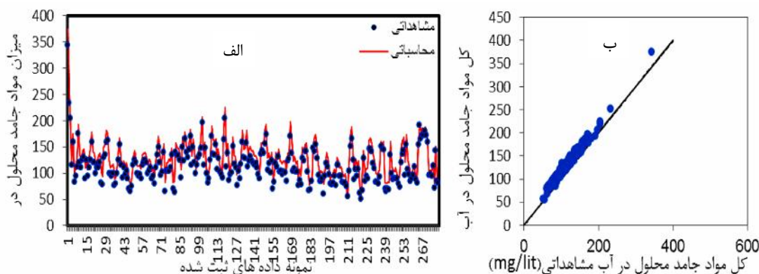
شکل ۶- نمودار حاصل از مقادیر بهینه مدل شبکه عصبی مصنوعی برای داده‌های ثبت شده مرحله صحت سنجی الف) مقادیر محاسباتی و مشاهداتی نسبت به زمان ب) نمودار پراکنش میان مقادیر مشاهداتی و محاسباتی
