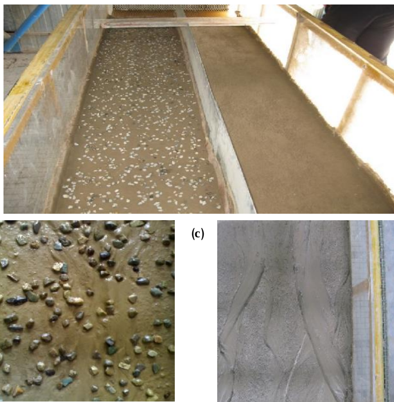
شکل ۱- (a) نمائی از فلوم مورد استفاده، (b) خاک بدون پوشش و (c) خاک ۳۰ درصد پوشش سنگ‌ریزه سطحی Figure 1. a) A schematic of flume used b) Soil with 0% surface cover c) Soil with 30% surface rock fragment cover
