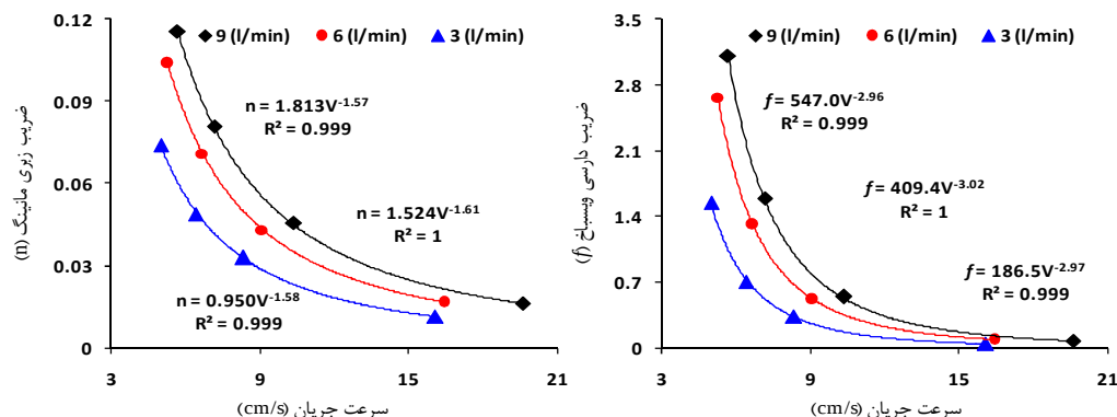
شکل ۴- رابطه بین ضرایب زبری مانینگ و دارسی وایسباخ با سرعت جریان سطحی Figure 4. Relation between Manning's and Darcy-Weisbach roughness coefficients surface flow velocity
