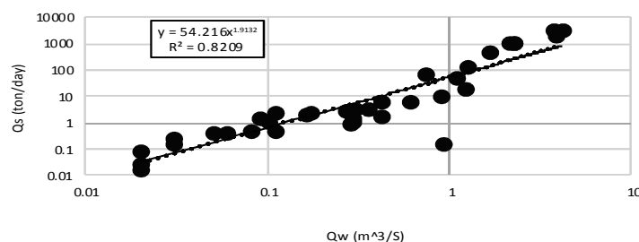
شکل ۲- منحنی سنجه رسوب زیر مدل ماه‌های فاقد پوشش گیاهی از مدل پوشش گیاهی در ایستگاه هیدرومتری گلستان جاغرق Figure 2. Sediment Rating Curve for "sub-model of months without of vegetation" from the vegetations model in hydrometric station of Golestan Jagharq
