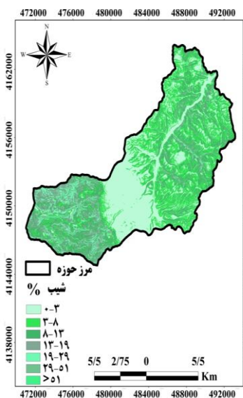
شکل ۵- نقشه شیب حوزه آبخیز روضة چای
