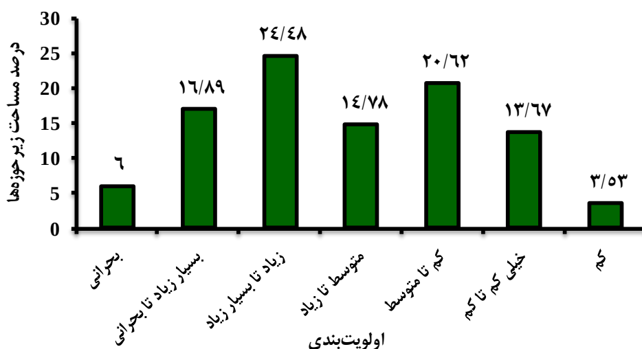
شکل ۶- اولویت‌بندی درصد مساحت زیرحوزه‌های آبخیز روضه‌چای براساس آنالیز مورفومتری
