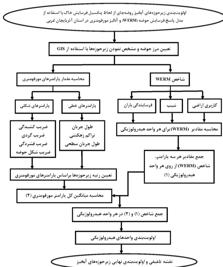
شکل ۲- نمودار جریانی اولویت‌بندی زیرحوزه‌ها با استفاده از مدل پاسخ فرسایش حوضه (WERM) و آنالیز مورفومتری Figure 2. The flowchart of sub-watersheds prioritization using Watershed Erosion Response Model (WERM) and morphometric analysis
