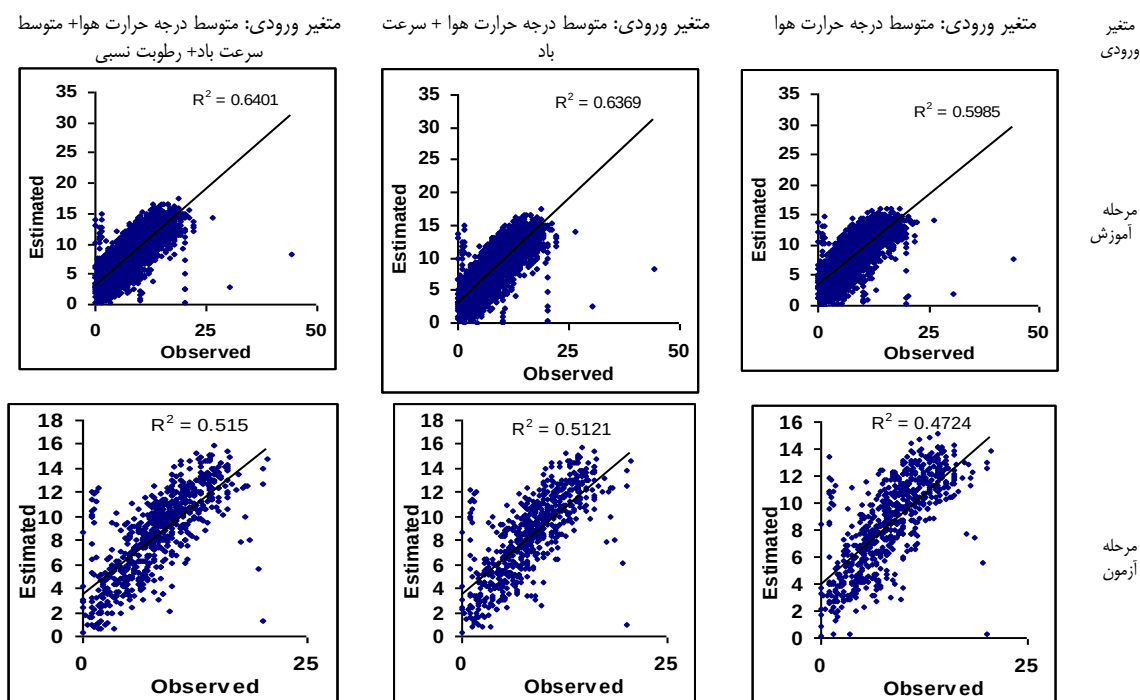
شکل ۶- Q-Q پلات مدل های بهینه رگرسیونی با متغیرهای ورودی مختلف Figure 6. Q-Q plot of optimal regression models with different input variables
