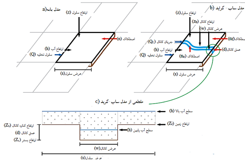
شکل ۲- شماتیکی از مدل LISFLOOD-FP: a: سلول‌های دشت سیلابی b: سلول‌های دشت سیلابی و کانال c: ارتباط بین سلول‌ها Figure 2. Model schematics for a. Floodplain only cell. b. Floodplain and channel cell c. interface between cells
