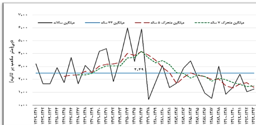
شکل ۴- تغییرات متوسط دبی سالانه ایستگاه کوپال نمره ۳ و میانگین متحرک ۷ و ۱۵ سال‌های طی سال‌های ۱۳۶۱ تا ۱۳۹۴ Figure4. Yearly variation of water flow rate average and its 7&15 years moving averages in Koopal No3 hydrometric station between the years of 1982-2014
