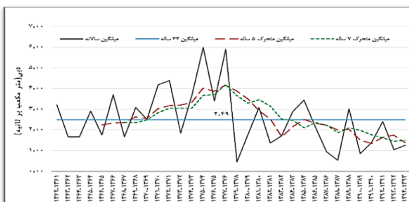
شکل ۴- تغییرات متوسط دبی سالانه ایستگاه کوپال نمره ۳ و میانگین متحرک ۷ و ۱۵ سال‌های طی سال‌های ۱۳۹۱ تا ۱۳۹۴ Figure4. Yearly variation of water flow rate average and its 7&15 years moving averages in Koopal No3 hydrometric station between the years of 1982-2014
