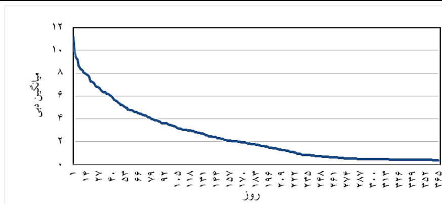
شکل ۵- منحنی تداوم جریان رودخانه کوپال بر اساس آمار ایستگاه آبسنجی کوپال نمره ۳ Figure 5. Flow duration curve of Koopal River based on the hydrometric station of the Koopal No 3
