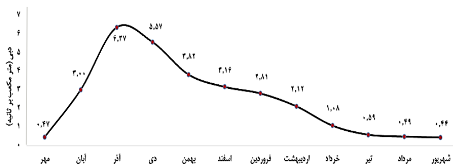
شکل ۲- تغییرات دبی متوسط ایستگاه کوپال بین سال های ۹۳-۹۴ تا ۶۲-۶۱
