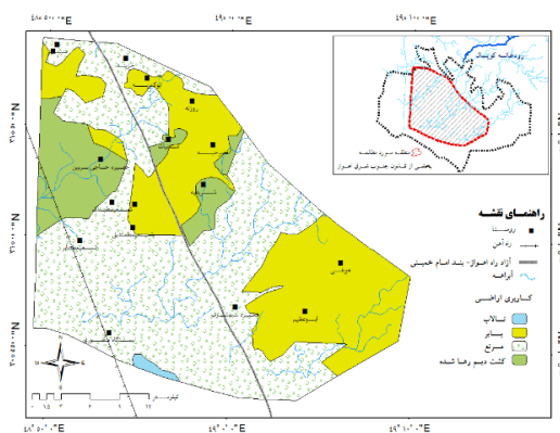
شکل ۱۰- نقشه کاربری اراضی محدوده Figure 10. Map of land use
