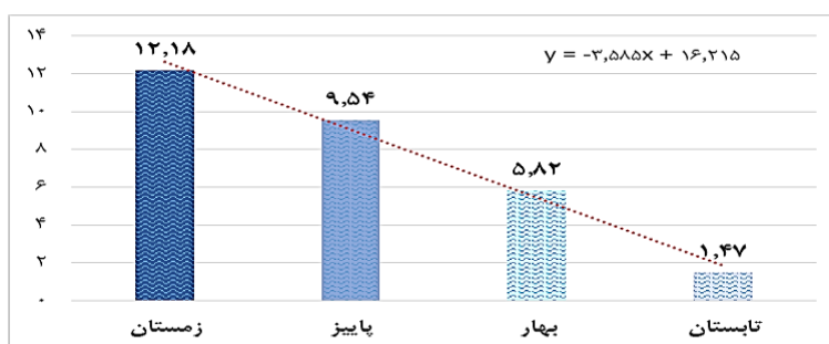
شکل ۳- تغییرات متوسط دبی فصلی ایستگاه کوپال نمره ۳ بین سال‌های آبی ۹۴-۹۳ تا ۶۲-۶۱ Figure 3. Variation of average seasonal water flow rate in Koopal No3 hydrometric station between the years of 1982-2014
