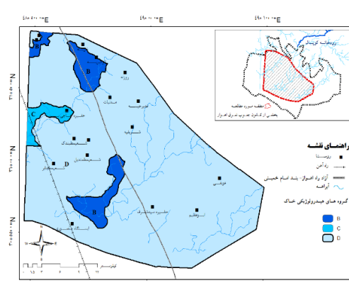
شکل ۹- نقشه گروه‌های هیدرولوژیکی خاک Figure 9. Map of soil hydrological groups
