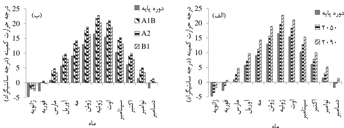
شکل ۲- الف: مقایسه میانگین ماهانه دمای کمینه ایستگاه میان‌دواب بر اساس سناریو A2 در سه دوره. ب: مقایسه میانگین ماهانه دمای کمینه ایستگاه میان‌دواب در دوره پایه و دوره ۲۰۹۰ بر اساس سه سناریو A1B، A2 و B1
