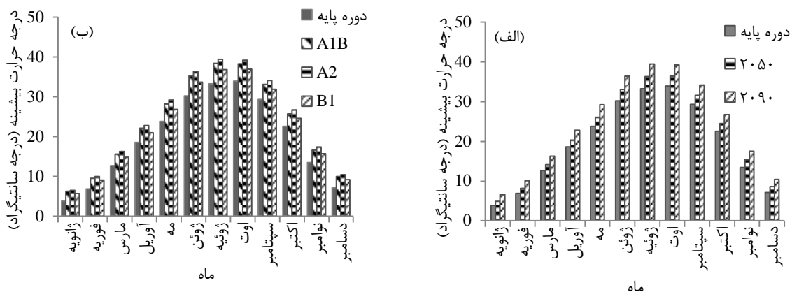
شکل ۳- الف: مقایسه میانگین ماهانه دمای بیشینه ایستگاه میان‌دواب بر اساس سناریو A2 در سه دوره. ب: مقایسه میانگین ماهانه دمای بیشینه ایستگاه میان‌دواب در دوره پایه و دوره ۲۰۹۰ بر اساس سناریو های A1B و A2 و B1
