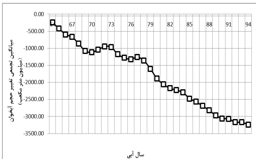
شکل ۲- تغییرات تجمعی حجم آبخوان دشت مشهد در بازه سال‌های ۱۳۶۴-۱۳۹۵ Figure 2. Cumulative changes in the size of Mashhad aquifer between 1964-1953
