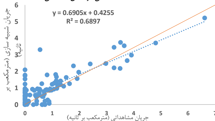
شکل ۱۰- همبستگی جریان مشاهداتی و شبیه‌سازی (واسنجی) در ایستگاه قاسملو Figure 9. Correlation of observation and simulation (calibration) flow at Ghasemlou Station
