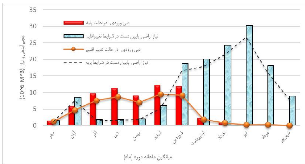
شکل ۳- میانگین ماهانه حجم آبدهی به مخزن به‌همراه میانگین ماهانه حجم تقاضای آب در شرایط پایه و تغییر اقلیم Figure 3. Average monthly inflow and water demand volume under baseline and climate change conditions
