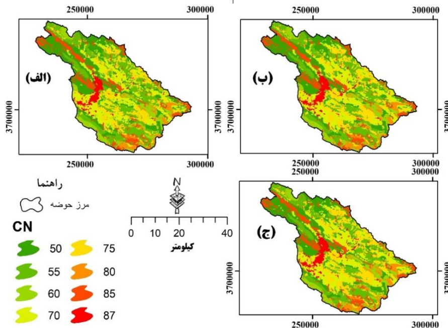
شکل ۴- تغییرات شماره منحنی در آبخیز خرم‌آباد در دوره مطالعاتی سال‌های ۲۰۱۱، ۲۰۱۹ و ۲۰۰۳ Figure 4. The trend in curve number of the Khorramabad watershed in the years 2003, 2011 and 2019
