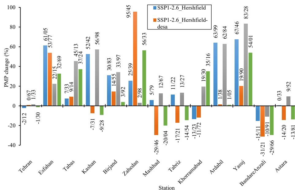
شکل ۶- درصد تغییرات PMP در آینده (۲۰۲۱-۲۰۴۰) نسبت به دوره پایه (۱۹۹۳-۲۰۲۲) در ایستگاه‌های همدید ایران Figure 6. The percentage of PMP changes in the future (2040-2021) compared to the base period (1993-2022) at the synoptic stations in Iran
