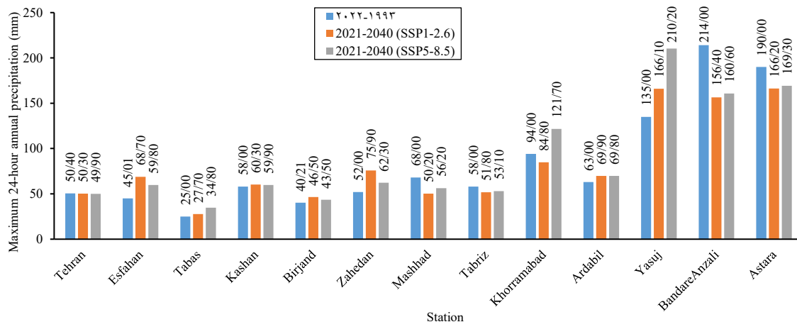
شکل ۴- حداکثر بارش ۲۴ ساعته سالانه (میلی‌متر) ایستگاه‌های هم‌مدید ایران تحت سناریوهای SSP1-2.6 و SSP5-8.5 در دوره پایه (۱۹۹۳-۲۰۲۲) و آینده (۲۰۲۱-۲۰۴۰)
