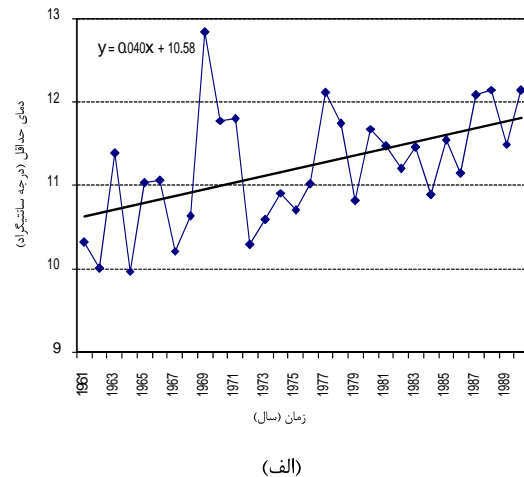
شکل ۲- الف) دمای کمینه و ب) دمای بیشینه ایستگاه یزد در دوره پایه ۱۹۶۱-۱۹۹۰.
