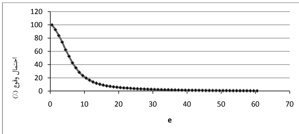
شکل ۲- منحنی تداوم جریان درازمدت سالانه رودخانه بابلرود- ایستگاه قرآن تالار دبی جریان (m³/s)
