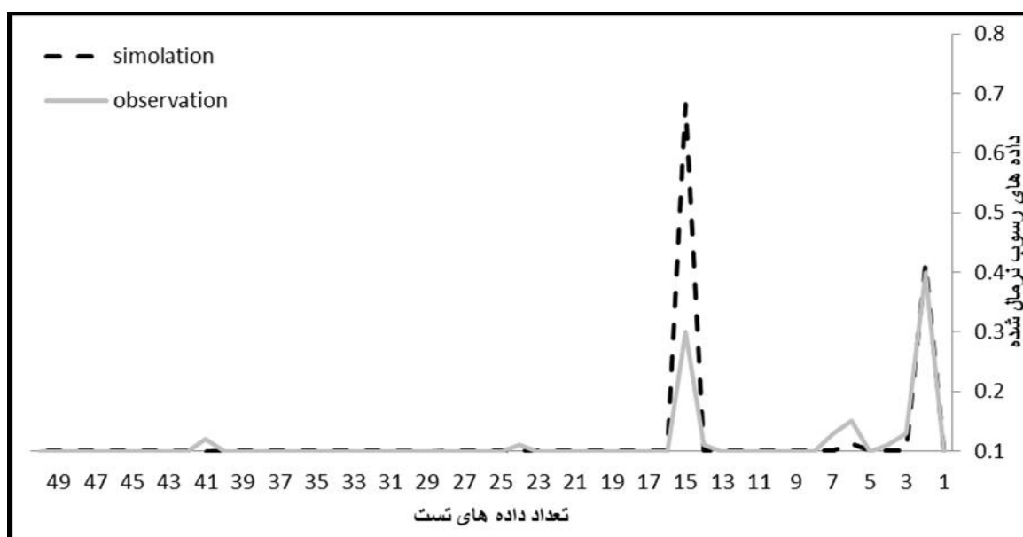
شکل ۴- مقایسه بین داده‌های اندازه‌گیری شده و شبیه‌سازی شده با مناسب‌ترین الگوریتم لونبرگ مارکوآرت (LM) به عنوان نمونه به منظور برآورد میزان رسوب در شبکه Cascade Forward back prop ایستگاه چم انجیر
