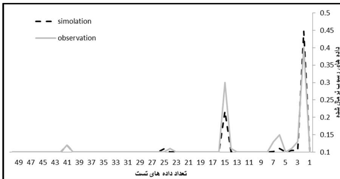
شکل ۳- مقایسه بین داده‌های اندازه‌گیری شده و خروجی مدل (شبیه‌سازی شده) با مناسب‌ترین الگوریتم لونبرگ مارکوآرت (LM) به عنوان نمونه برای برآورد میزان رسوب در شبکه fitting ایستگاه چم انجیر
