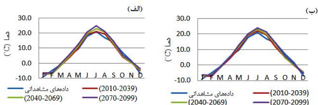
شکل ۸- مقایسه دمای کمینه ماهانه مشاهداتی و شبیه‌سازی شده شهر بم توسط سناریو A2 (الف) و B2 (ب)
