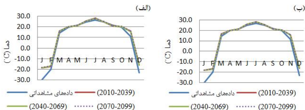
شکل ۵- مقایسه دمای کمینه ماهانه مشاهداتی و شبیه‌سازی شده شهر کرمان توسط سناریو A2 (الف) و B2 (ب)
