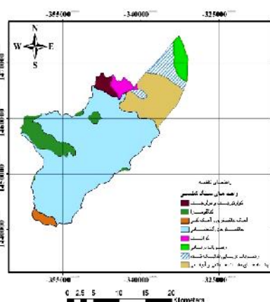
شکل ۳- نقشه واحدهای سنگ‌شناسی در حوزه آبخیز شلمانرود
