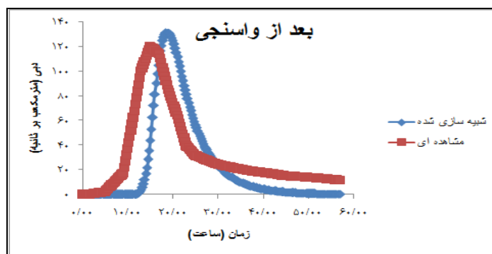
شکل (۴-۱۸) سیلاب مورخ ۱۳۶۹/۱۰/۱۲ بعد از واسنجی.
