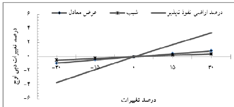
شکل ۴- درصد تغییرات عرض معادل، شیب و درصد اراضی نفوذناپذیر و تاثیر آن بر دبی اوج برحسب درصد.
