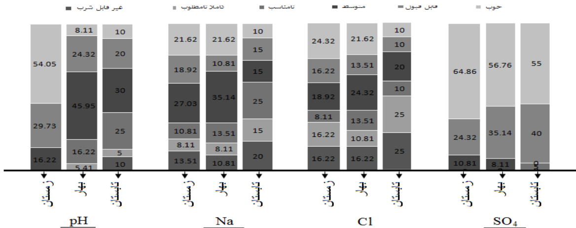
شکل ۵- درصد کلاس‌های طبقه‌بندی شولر برای مصارف آب شرب در فصل زمستان Figure 5. Percent for Schuler classifications for domestic water consumption in winter
