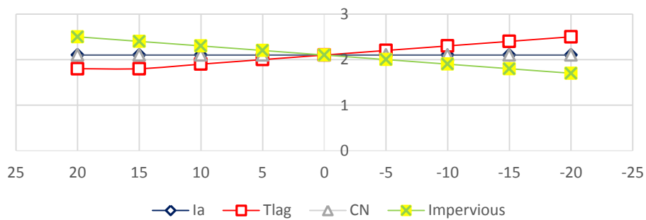
شکل ۵- تحلیل حساسیت پارامترها در حوزه یکپارچه کوه سوخته، (رویداد ۹۱/۱۰/۰۱)
