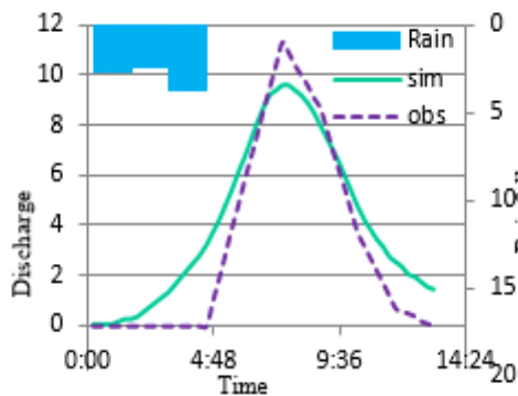
شکل ۶- دبی مشاهده‌ای و شبیه‌سازی شده در رویداد ۹۰/۱۱/۱۲ در حوزه نیمه‌توزیعی کوه‌سوخته-زیر حوزه ۱ Fig. 6. Observational and simulated discharge in the event of 2012/2/1 in the semi-distributive Kohsukhteh watershed-sub-catchment 1
