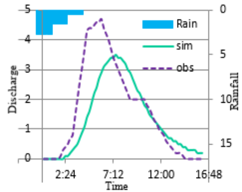
شکل ۱۱- دبی مشاهده‌ای و شبیه‌سازی شده در رویداد ۹۱/۱۰/۰۵ در حوزه یکپارچه کوه‌سوخته Fig. 11. Observational and simulated discharge in the event of 2012/12/25 in the Lumped Kohsukhteh watershed .
