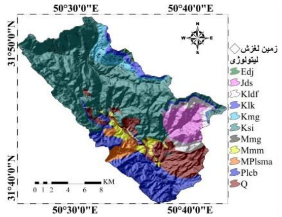
شکل ۲- لیتولوژی Figure 2. Lithology
