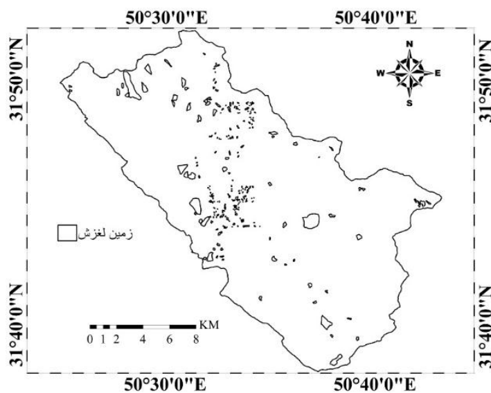
شکل ۱۴- نقشه پراکنش زمین لغزش Figure 14. Landslide inventory map
