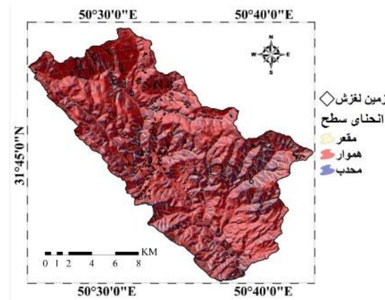
شکل ۱۲- انحنای سطح Figure 12. Plan curvature
