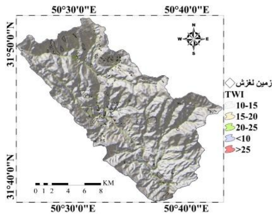
شکل ۱۱- شاخص خیسگی توپوگرافی Figure 11. Topography wetness index
