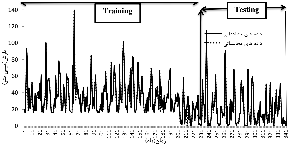
شکل ۷- الف و ب) مقادیر مشاهده‌ای و پیش‌بینی شده بارش ایستگاه سینوپتیک تبریز با شبکه بیزین و رگرسیون خطی چندمتغیره (ترکیب ۳) بخش آموزش و صحت سنجی
