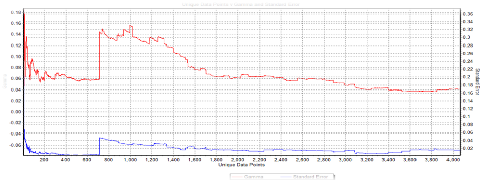
شکل ۴- آزمون M مقادیر گاما برای مدل منتخب در ایستگاه رشت Figure 4. M test of the selection Model on Rasht station
