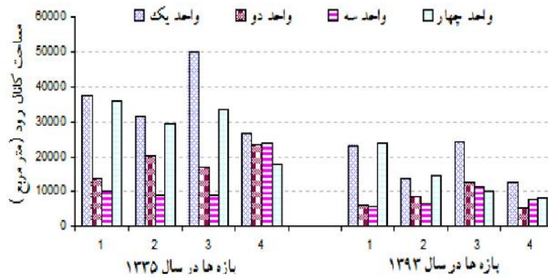
شکل ۳- تغییرات مساحت آبراه به تفکیک بازه‌های چهارگانه در سال‌های ۱۳۹۳-۱۳۳۵ Figure 3. Changes in the channel area in four-site intervals during 1956-2014
