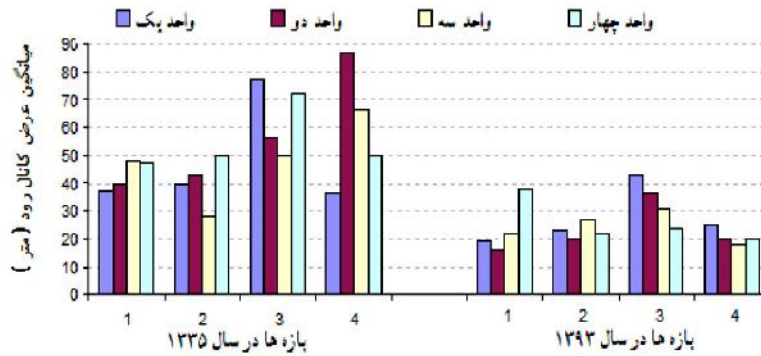
شکل ۴- تغییرات عرض آبراه رود طی سال‌های ۱۳۹۳-۱۳۳۵ Figure 4. Changes in the width of the river channel during 1956-2014
