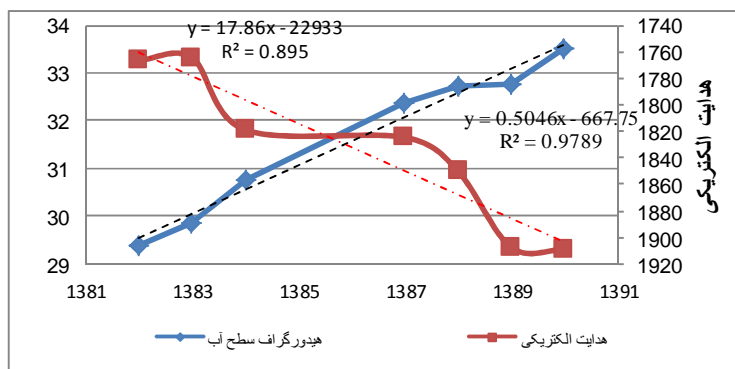
شکل ۹- رابطه هیدروگراف واحد سطح آب زیرزمینی و متوسط هدایت الکتریکی در دشت مرند
