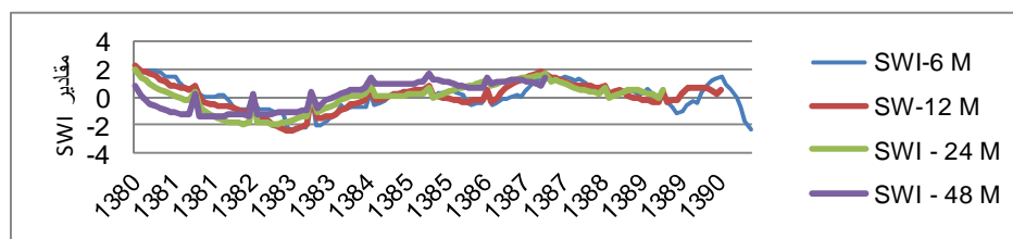
شکل ۳- وضعیت خشکسالی‌ها و ترسالی‌های پیزومتر نمونه (قره قوم) در مقیاس‌های زمانی مختلف Figure 3. Condition of Droughts and Wetness Sample piezometers (Ghareh Ghom) in different time scales
