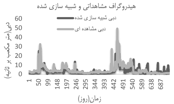
شکل ۱۱- هیدروگراف مشاهداتی و شبیه‌سازی شده برای دوره اعتبارسنجی (مقیاس ماهانه، ۱۳۸۷-۱۳۸۹) Figure 11. Observed and simulated hydrograph of validation (Monthly scale, 1387-1389)
