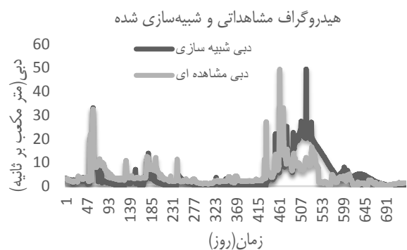
شکل ۱۳- هیدروگراف مشاهداتی و شبیه‌سازی شده برای دوره اعتبارسنجی (مقیاس سالانه، ۱۳۸۷-۱۳۸۹) Figure 13. Observed and simulated hydrograph of validation (Annual scale, 1387-1389)
