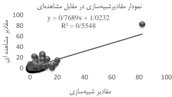
شکل ۴- مقایسه دبی متوسط روزانه مشاهداتی و شبیه‌سازی شده برای دوره واسنجی (مقیاس روزانه ۱۳۸۵-۱۳۸۷) Figure 4. Compare observed and simulated average daily flow of calibration (Daily scale, 1385-1387)
