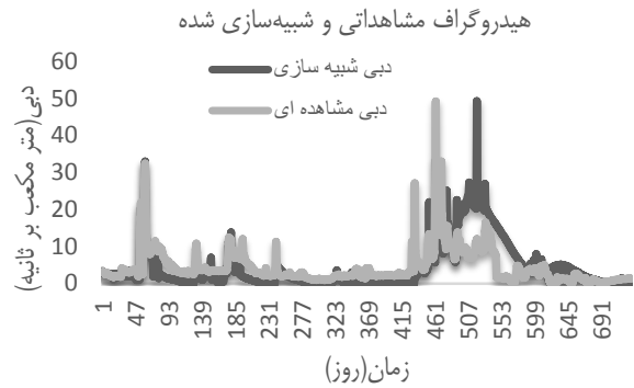
شکل ۹- هیدروگراف مشاهداتی و شبیه‌سازی شده برای دوره اعتبارسنجی (مقیاس روزانه، ۱۳۸۷-۱۳۸۹) Figure 9. Observed and simulated hydrograph of validation (Daily scale, 1387-1389)
