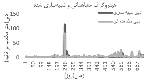
شکل ۵- هیدروگراف مشاهداتی و شبیه‌سازی شده برای دوره واسنجی (مقیاس ماهانه ۱۳۸۵-۱۳۸۷) Figure 5. Observed and simulated hydrograph of calibration (Monthly scale, 1385-1387)
